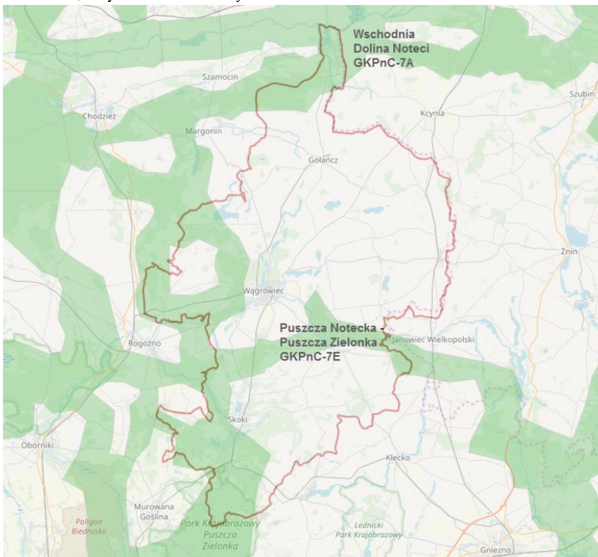
Ryc. 24. Przebieg korytarzy ekologicznych wg Instytutu Biologii Ssaków Polskiej Akademii Nauk Białowieża wg projektu 2005
